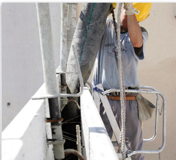
bétonnage
